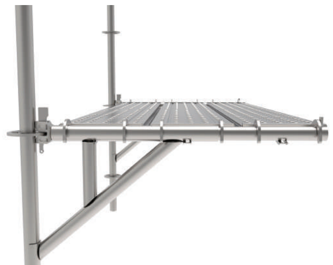
3塊踏板圖示
