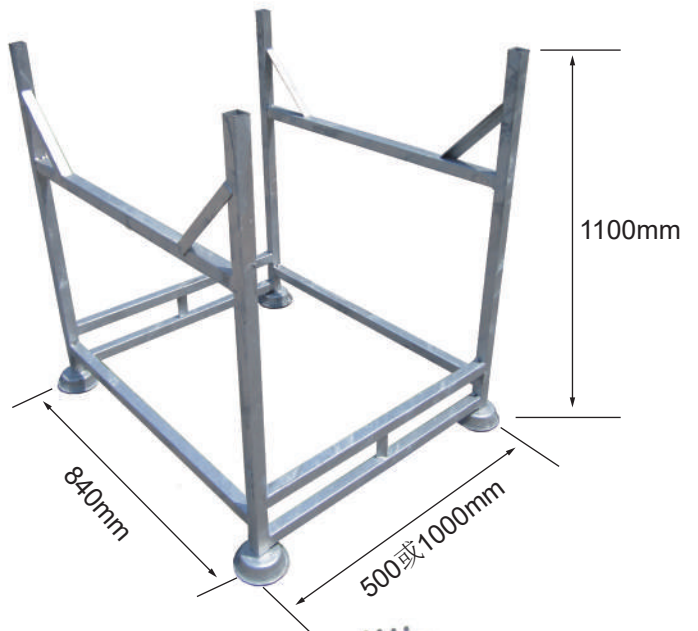
吊車吊運
